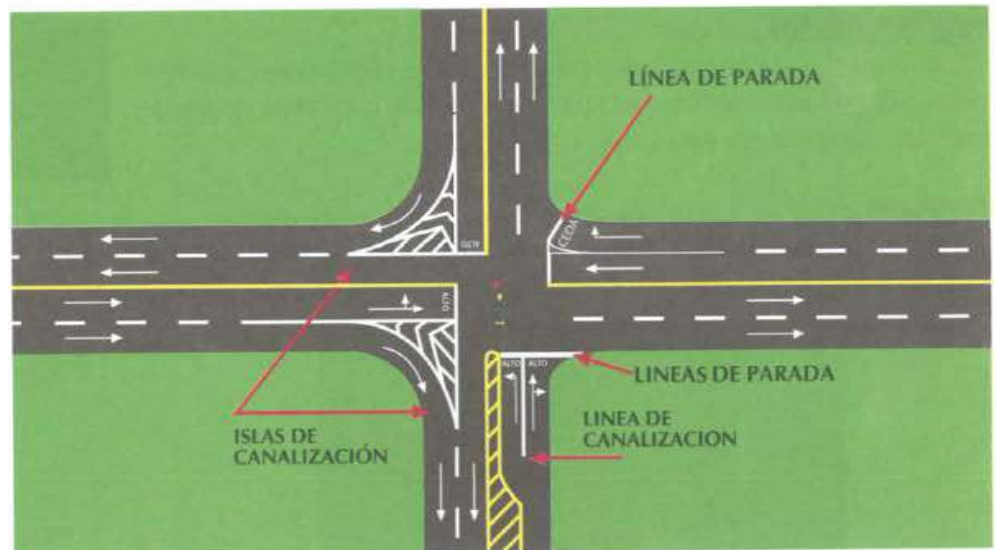
GRÁFICO 14: Intersección con sus componentes de regulación.
