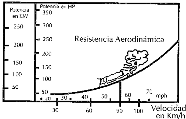
Resistencia aerodinámica
